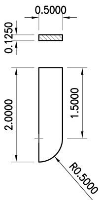
Fan Blade Detail
